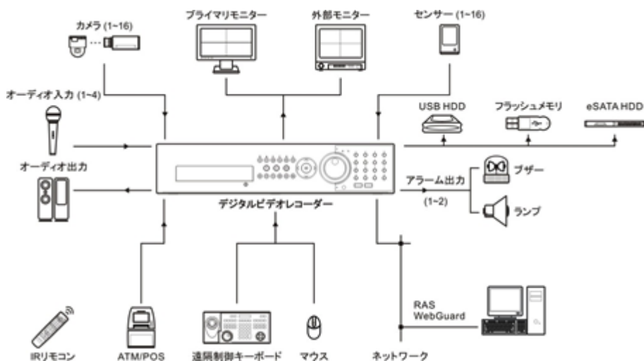
図1:サンプル構成図
