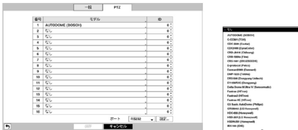
図39:カメラ / PTZ設定画面
