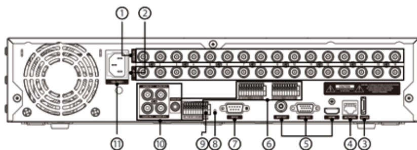
図2:16チャンネルDVR背面パネル
