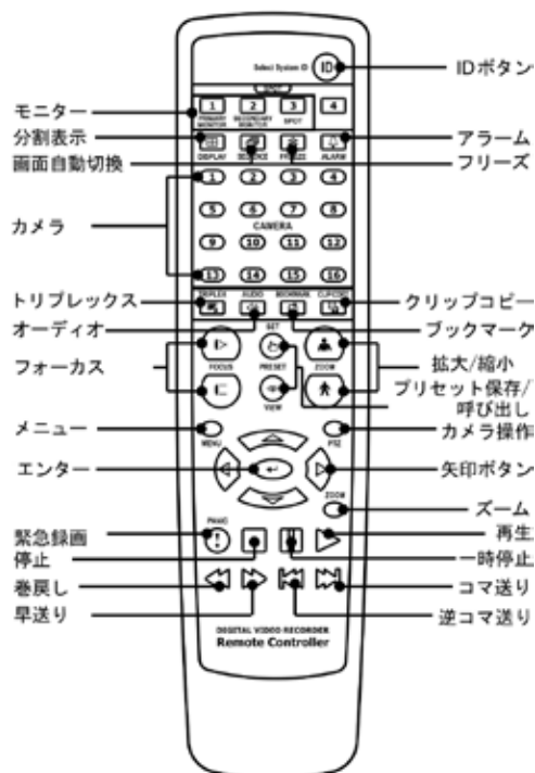
図4:IRリモコン
